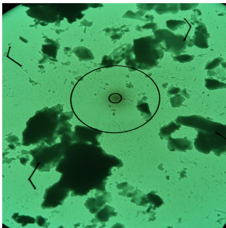
Obr. 1 Mikrofoto TEM vz. 16896/66/sp, úlomky horniny. Zvětšeno 2500x, průměr vnitřního terče je 1,9 \mu\text{m} .
