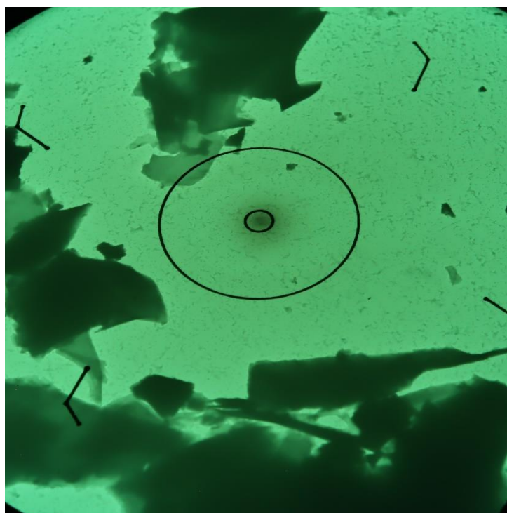
Obr. 1 Mikrofoto TEM vz. 16896/66/kr, úlomky horniny. Zvětšeno 2500x, průměr vnitřního terče je 1,9 \mu\text{m} .
