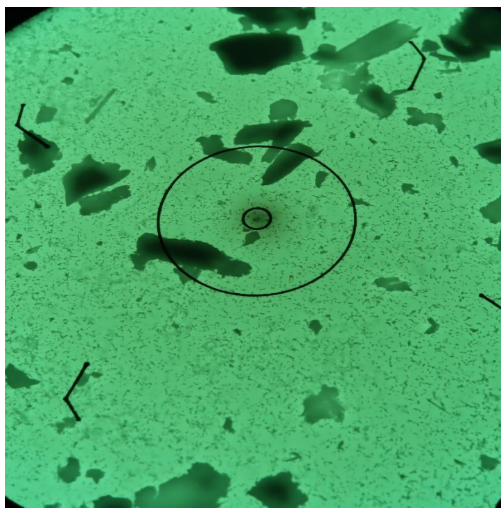
Obr. 1 Mikrofoto TEM vz. 16953/69, úlomky horniny. Zvětšeno 2500x, průměr vnitřního terče je 1,9 \mu\text{m} .
