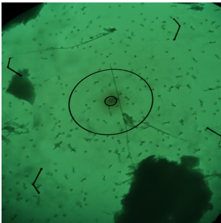
Obr. 2 Mikrofoto TEM vz. 16894/63, azbestová vlákna. Zvětšeno 13500x, průměr vnitřního terče je 0,4 \mu\text{m} .
