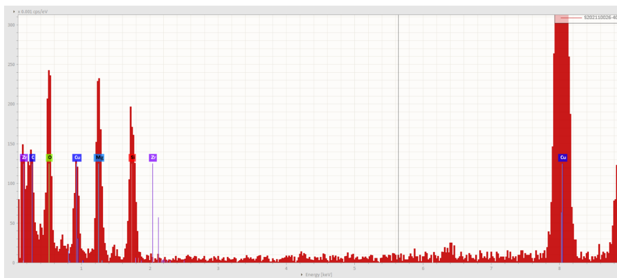
Obr. 3 EDS spektrum chryzotilového azbestového vlákna, vz. 16894/63.
