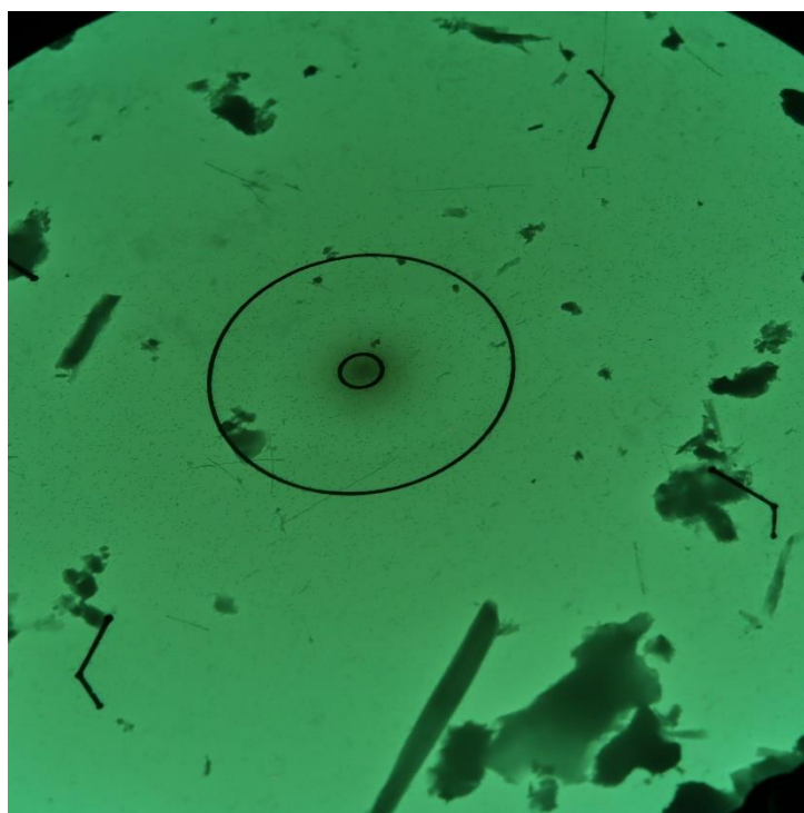
Obr. 1 Mikrofoto TEM vz. 16894/63, úlomky horniny. Zvětšeno 2500x, průměr vnitřního terče je 1,9 \mu\text{m} .
