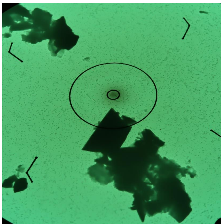
Obr. 1 Mikrofoto TEM vz. 16893/21, úlomky horniny. Zvětšeno 2500x, průměr vnitřního terče je 1,9 \mu\text{m} .
