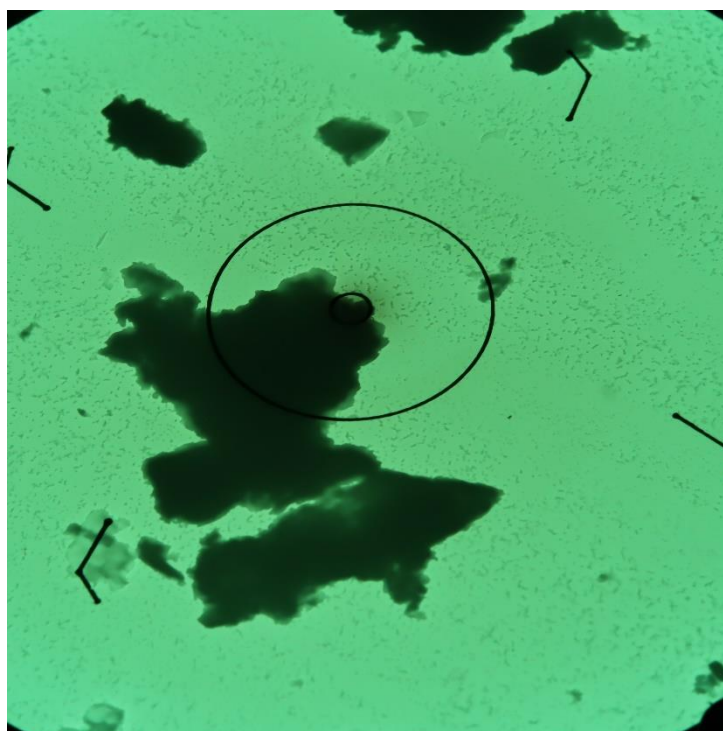
Obr. 1 Mikrofoto TEM vz. 17197/58, úlomky horniny. Zvětšeno 2500x, průměr vnitřního terče je 1,9 \mu\text{m} .
