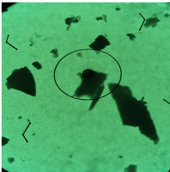
Obr. 1 Mikrofoto TEM vz. 16958/32, úlomky horniny. Zvětšeno 2500x, průměr vnitřního terče je 1,9 \mu\text{m} .
