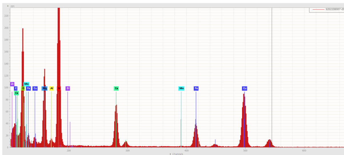
Obr. 3 EDS spektrum aktinolitového azbestového vlákna, vz. 17012/1.
