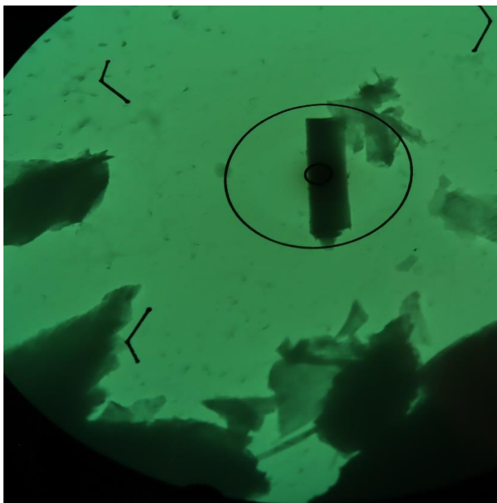
Obr. 2 Mikrofoto TEM vz. 16976/73, azbestová vlákna. Zvětšeno 13500x, průměr vnitřního terče je 0,4 \mu\text{m} .
