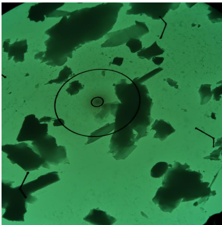
Obr. 1 Mikrofoto TEM vz. 16976/73, úlomky horniny. Zvětšeno 2500x, průměr vnitřního terče je 1,9 \mu\text{m} .
