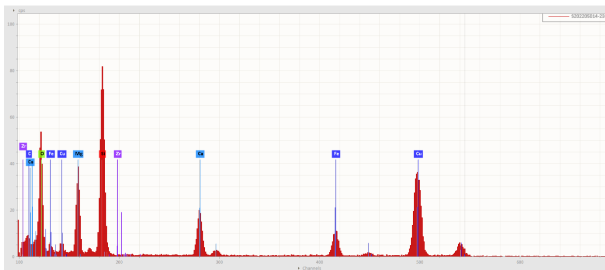
Obr. 3 EDS spektrum aktinolitového azbestového vlákna, vz. 16976/73.
