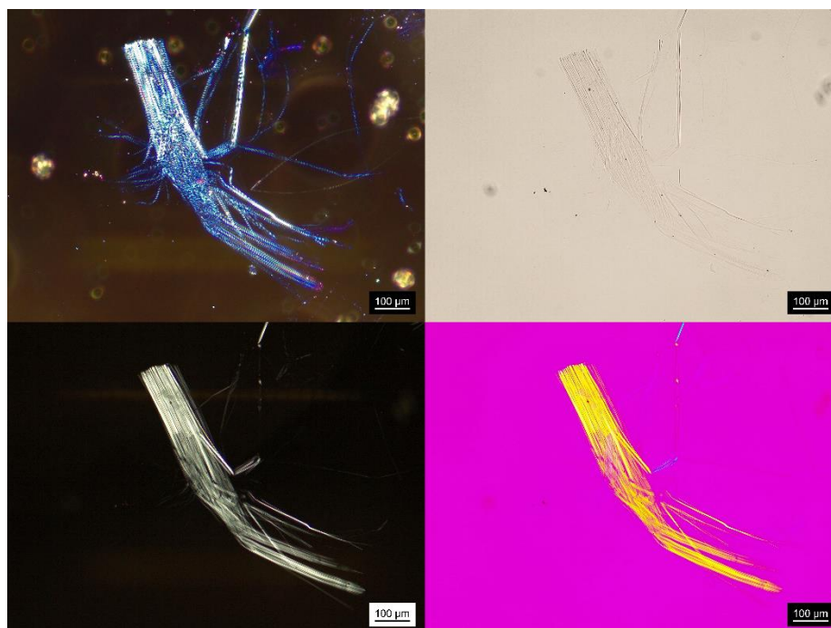
Obr. 1 Mikrofoto OPM vz. 16951/26, azbestová vlákna (ve směru čtení postupně: objektiv disperzního barvení, rovnoběžné polarizátory, zkřížené polarizátory, zkřížené polarizátory s destičkou fázového posunu 530 nm).
