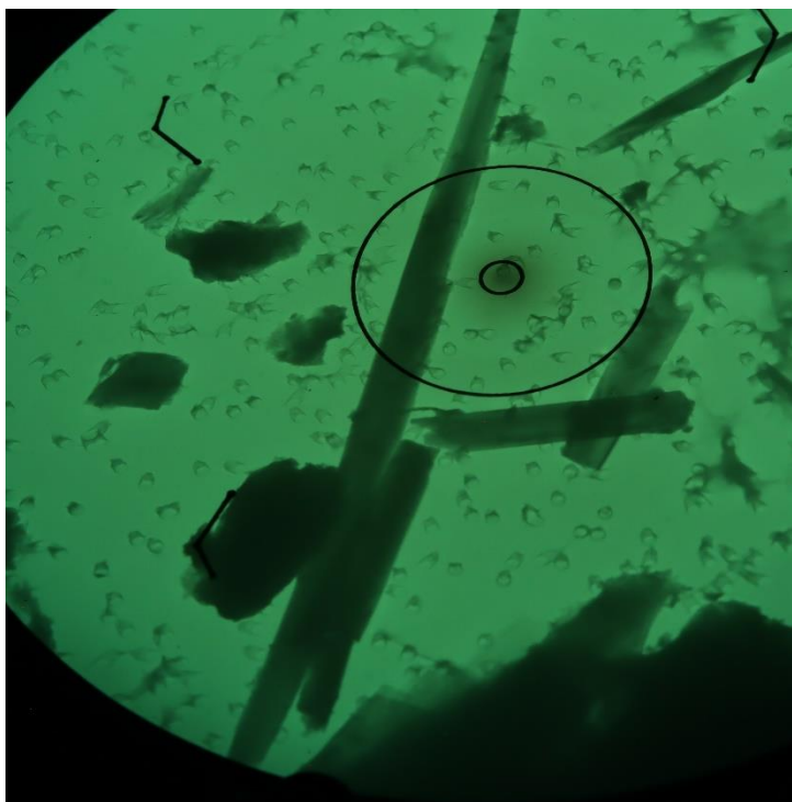
Obr. 2 Mikrofoto TEM vz. 16883/82, azbestová vlákna. Zvětšeno 13500x, průměr vnitřního terče je 0,4 \mu\text{m} .
