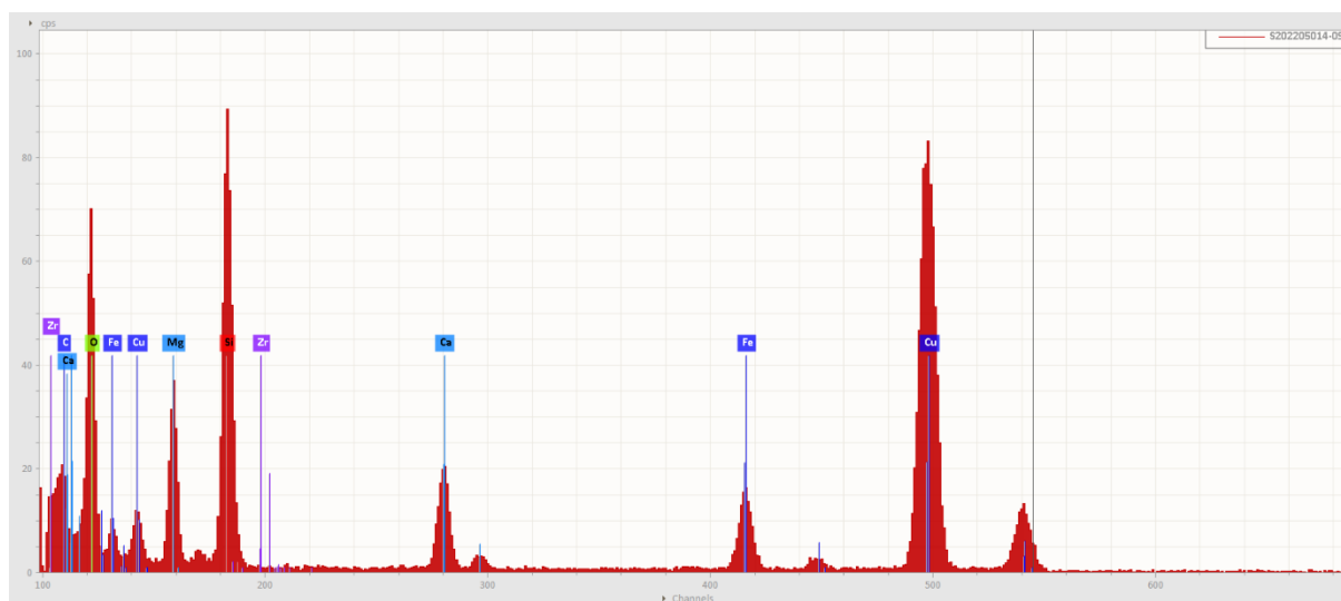
Obr. 3 EDS spektrum aktinolitového azbestového vlákna, vz. 16883/82.
