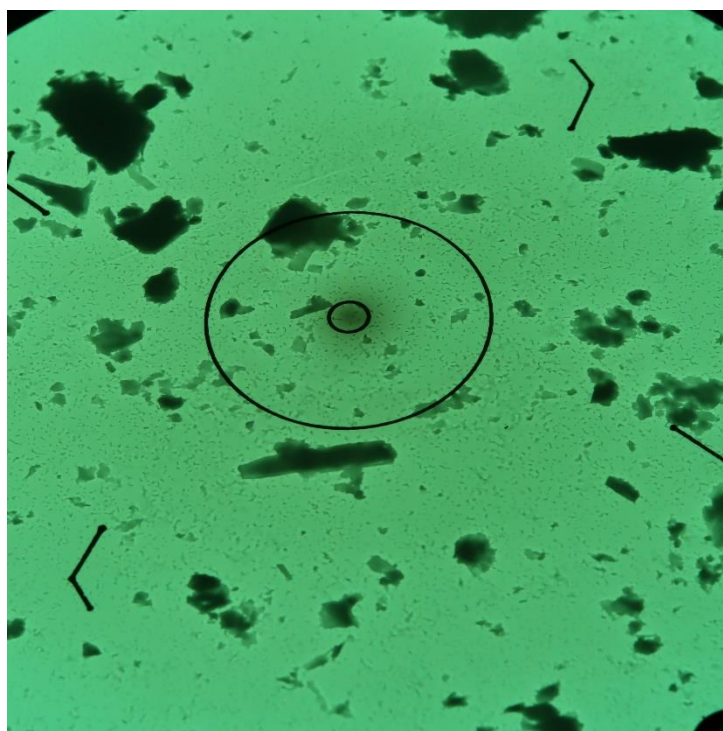
Obr. 1 Mikrofoto TEM vz. 16991/6, úlomky horniny. Zvětšeno 2500x, průměr vnitřního terče je 1,9 \mu\text{m} .
